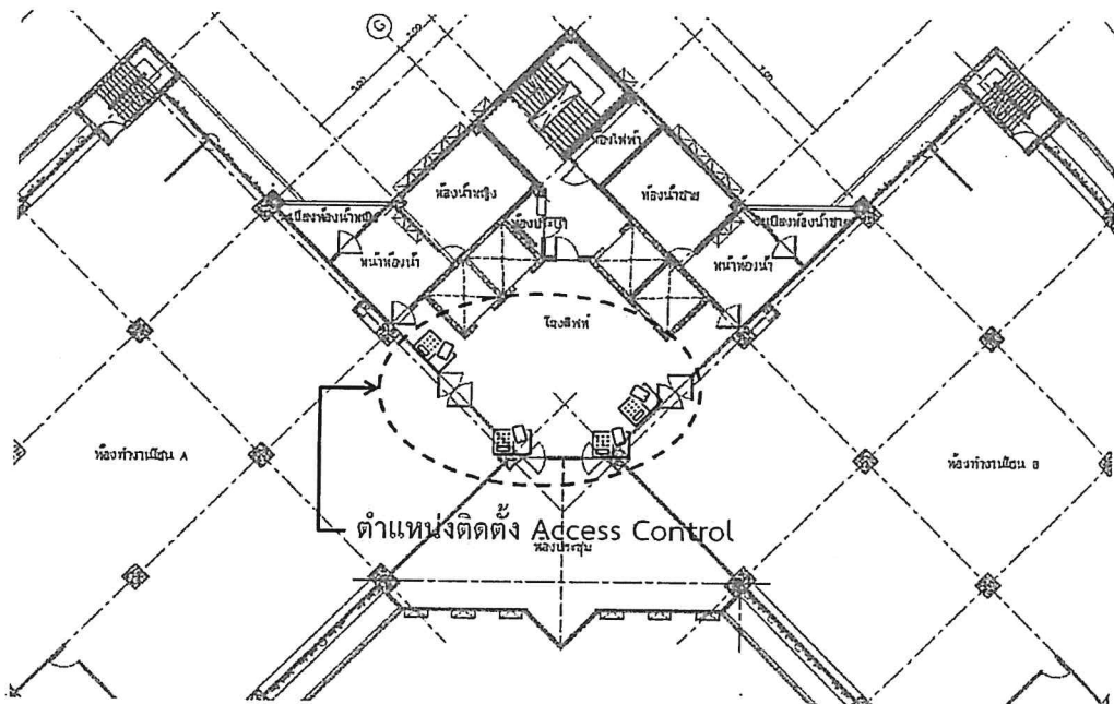
ตำแหน่งติดตั้งระบบ Access control ชั้น 3 - 4
